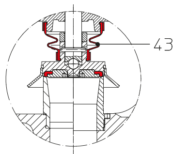
(Ausführung DN 20-100) (Ausführung DN125-150) EPDM-WEDI-Kegel, EPDM-Faltenbalg
