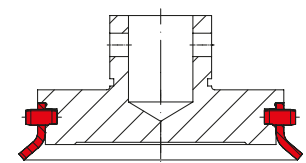
Berstscheibe (Auslegung siehe Seite 46.)
