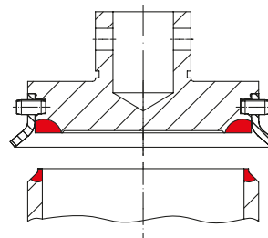
Sitz 1.4571 / Stellt No. 21 Kegel 1.4571 / Stellt No 6 Sitz SA479 Gr.316 Ti / Stellt No. 21 (SAFE-SN ANSI) Kegel SA479 Gr.316 Ti / Stellt No. 6 (SAFE-SN ANSI) und lösbare Hubhilfe
