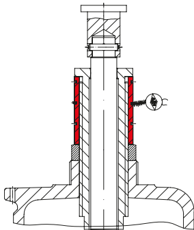
Sperrhülse
