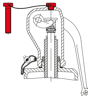
Blockierschraube
